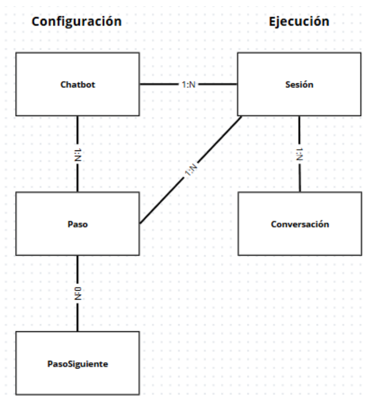
Diagrama ER
